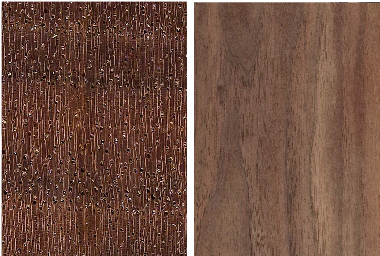
Nussbaum ( Juglans nigra .): Querschnitt (ca.12x) und tangentielle Oberfläche (natürliche Größe)
