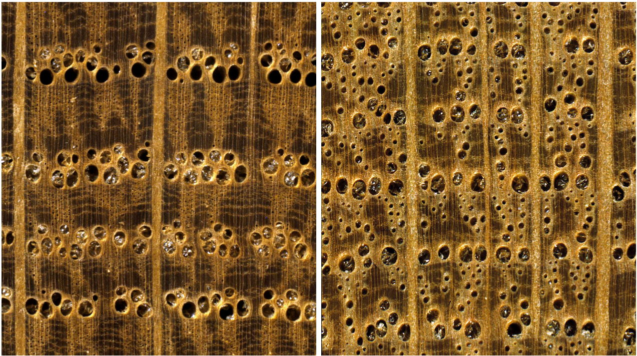
Holz vom Typ Weißeiche (links) und Roteiche (rechts) ( Quercus spp.) im Querschnitt (ca. 12x) mit deutlichem Unterschied in der Ausbildung der Spätholzporen
